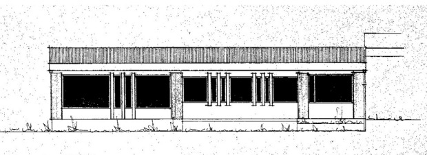
Skýringarmynd: Útlit vestur núverandi 1:250
