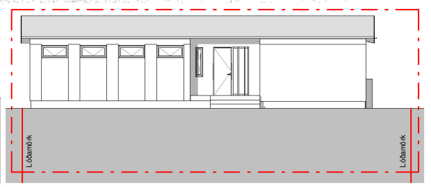
Skýringarmynd: Útlit austur núverandi 1:250
