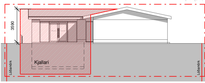
Skýringarmynd: Útlit suður tillaga að breytingu 1:250 Ekki til teikning af núverandi útlit suður.
